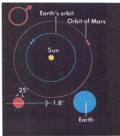
Mars in orbit
