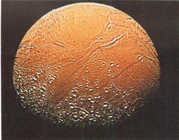
Enceladus NASA
