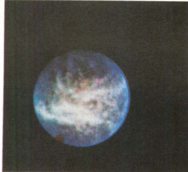
Rhea NASA
