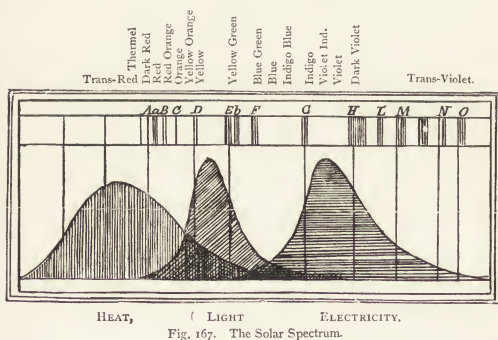
Fig. 167. The Solar Spectrum.
