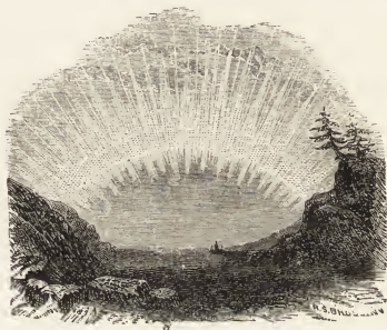
Fig. 96. The Aurora Borealis.
