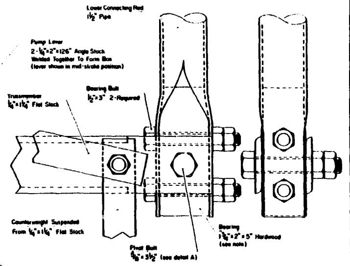
Lever End Pivot
