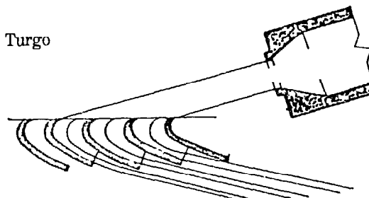
Figura 7b Contraste de las Turbinas Turgo y Pelton. El Chorro en la Turbina Turgo Golpea Continuamente Tres Cubos, Mientras que, en la Pelton, Sólo Golpea Uno. Un efecto Análogo de Incremento de la Velocidad Puede Obtenerse en la Turbina Pelton Añadiendo Uno o Dos Chorro Más.
