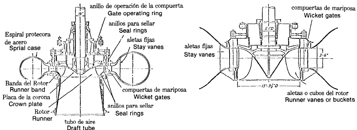
a) Turbina de reacción Allis-Chalmers, n_s = 26 .
