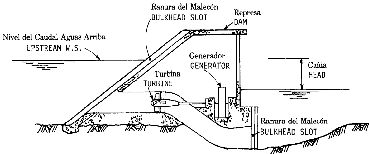
B) Instalación de una Turbina de Tubo B) TUBE-TURBINE INSTALLATION
