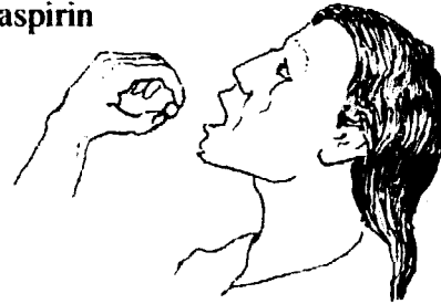
aspirin
