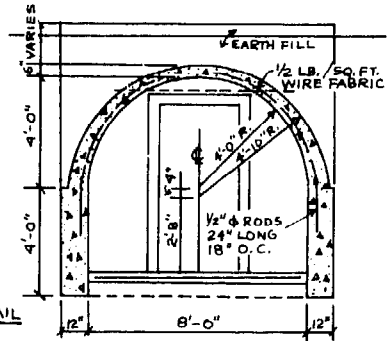
OPTIONAL SECTION A-A SCALE: 1/4" = 1'-0"
