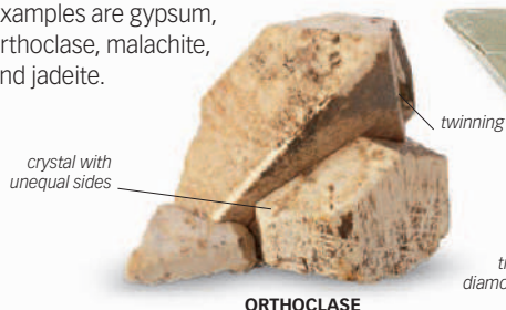
ORTHOCLASE
