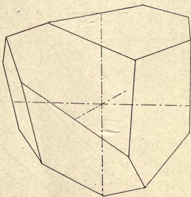
FIG. 42. +R \left( \frac{a:2a:3a}{4} \right) .
