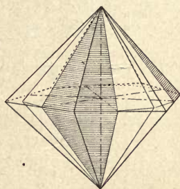
FIG. 191. — The Plus Ditrigonal Pyramid ( hkl ).
