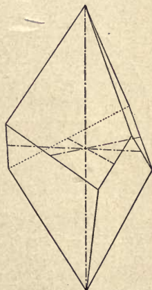
FIG. 209. — The Plus Left Trapezohedron.
