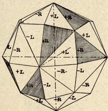
FIG. 41. ( a:2a:3a .)
