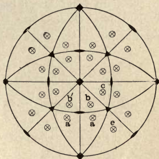
FIG. 73 a. — Hexoctahedron.
