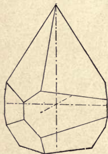
FIG. 145. — Wulfenite, (111) (11\bar{1}) (001) (430) .
