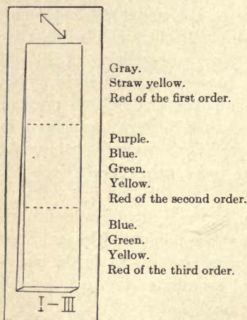
FIG. 334. — Quartz Wedge.
