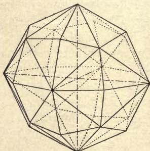
FIG. 73. — The Hexoctahedron, 3a : a : 2a .
