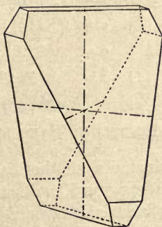
FIG. 235. — Sulphur.
