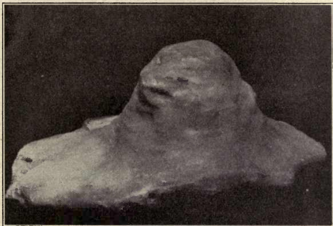
FIG. 391. — Stalagmite of Calcite.
