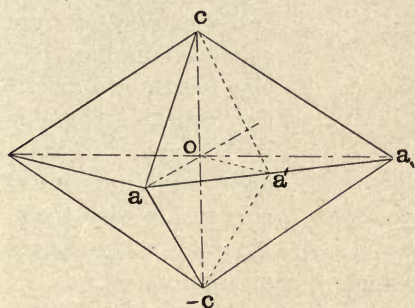
FIG. 148. — Cassiterite, (111).
