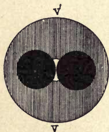
FIG. 303.—The Websky Signal.
