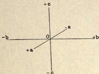
FIG. 20. — Crystallographical Axes.
