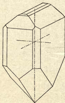
FIG. 231. — Calamine.
