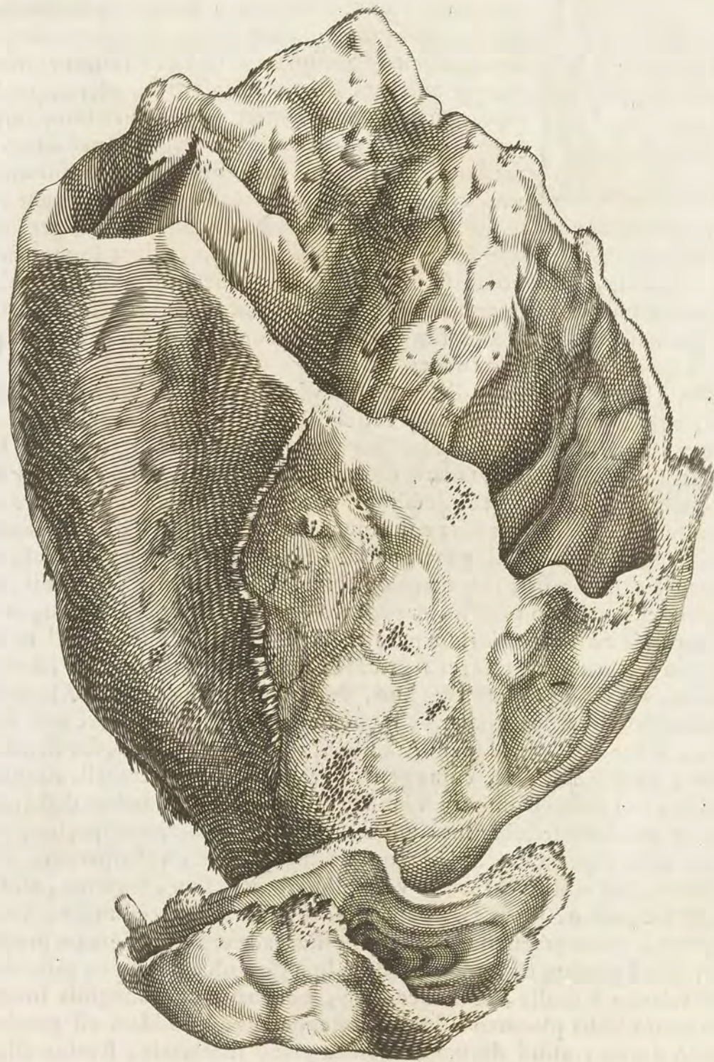
ALCYONIUM PRIMVM
