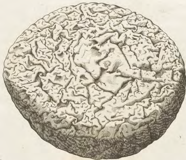
TOPHVS JUVENCARVM.
