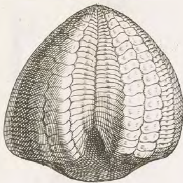
VERTEX
