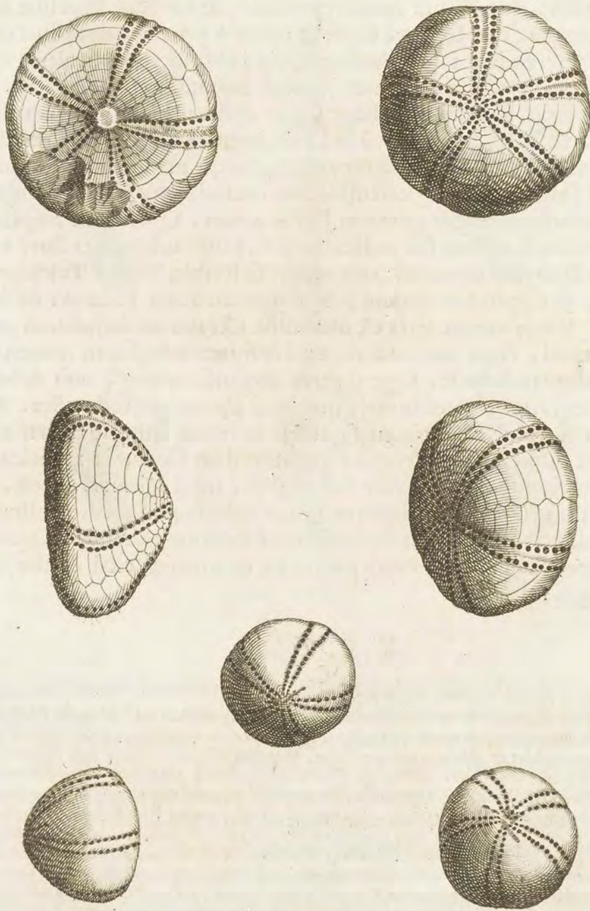
BRONTIA
