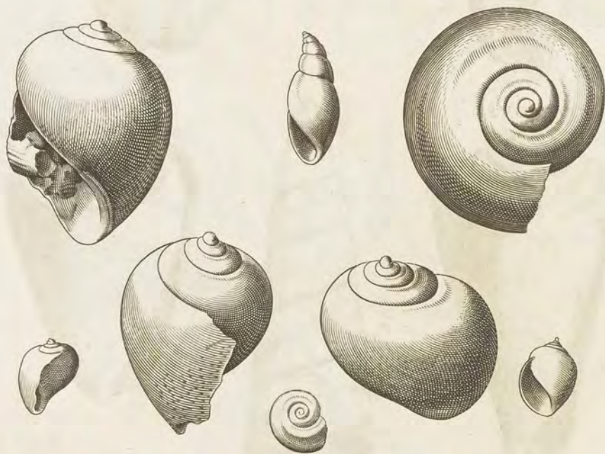
COCHLEA LAPIDEA
