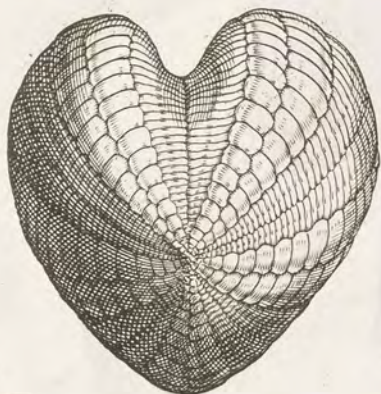
VERTEX
