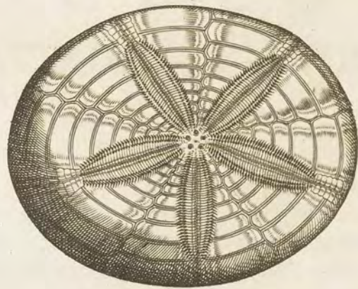
MONOSTROITES
