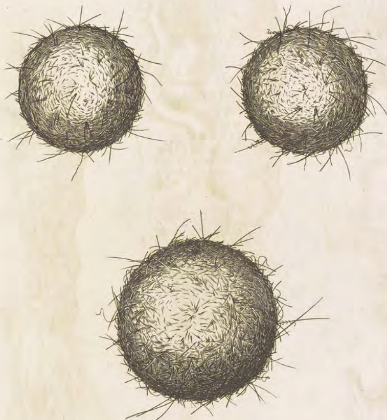
PILA MARINA
