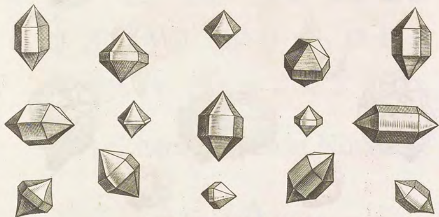
LAPIS DICONVS
