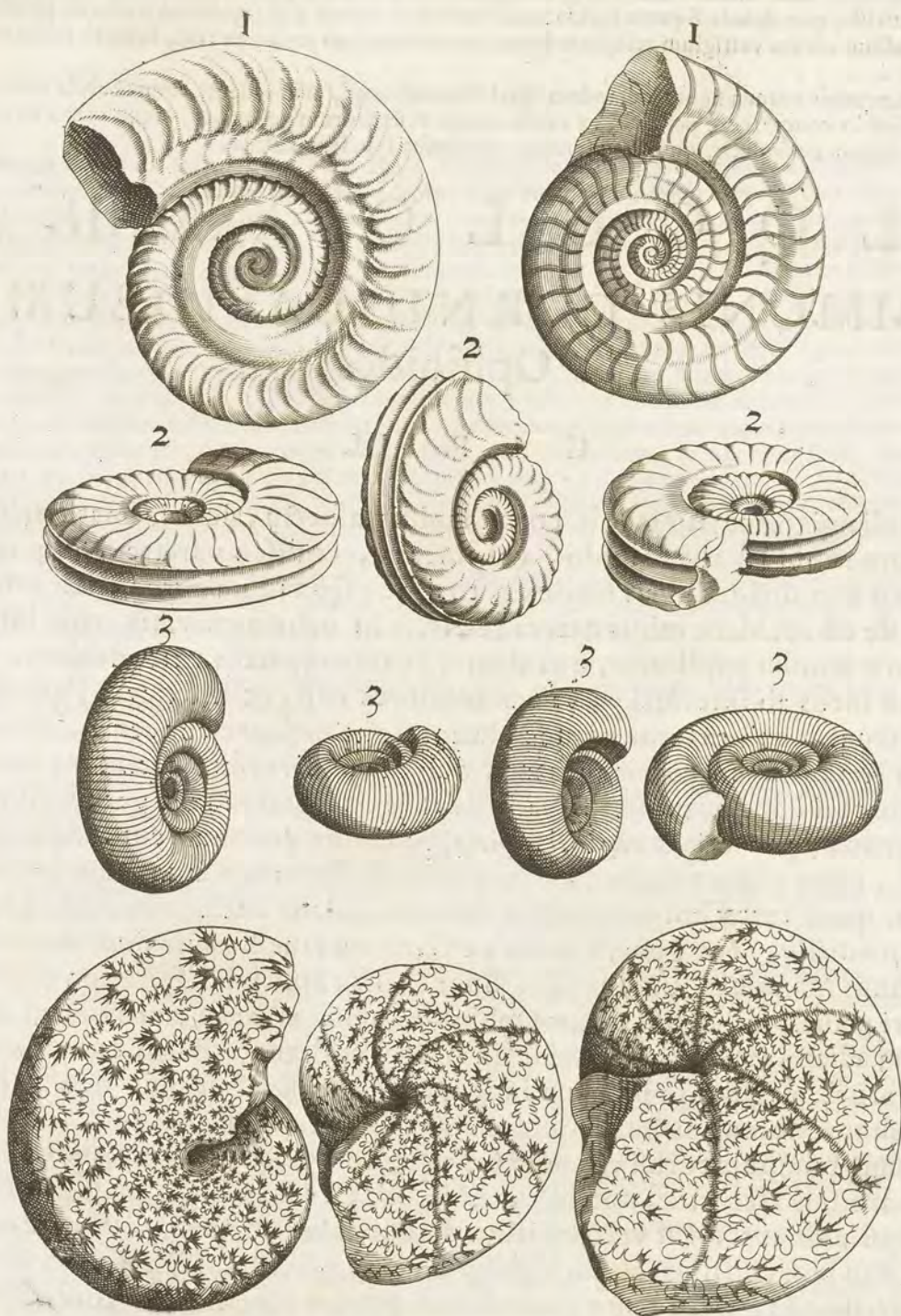
OPHIOIDES
