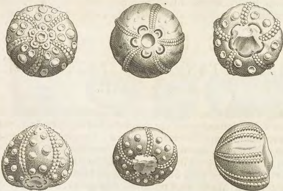
SCOLOPENDRITES LAPIS
