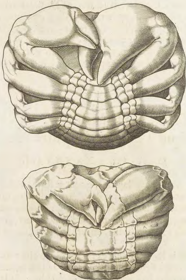
CANCER LAPIDEVS
