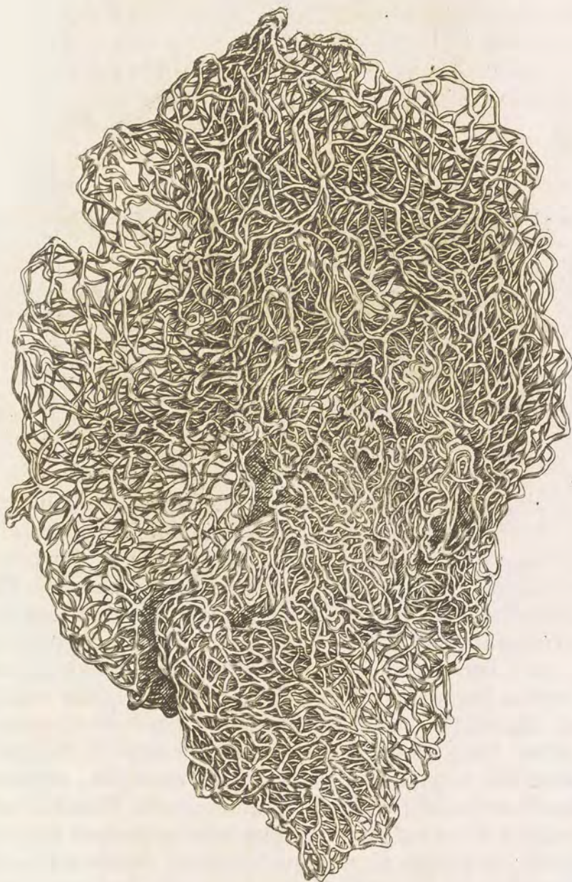
ALCYONIVM TERTIVM
