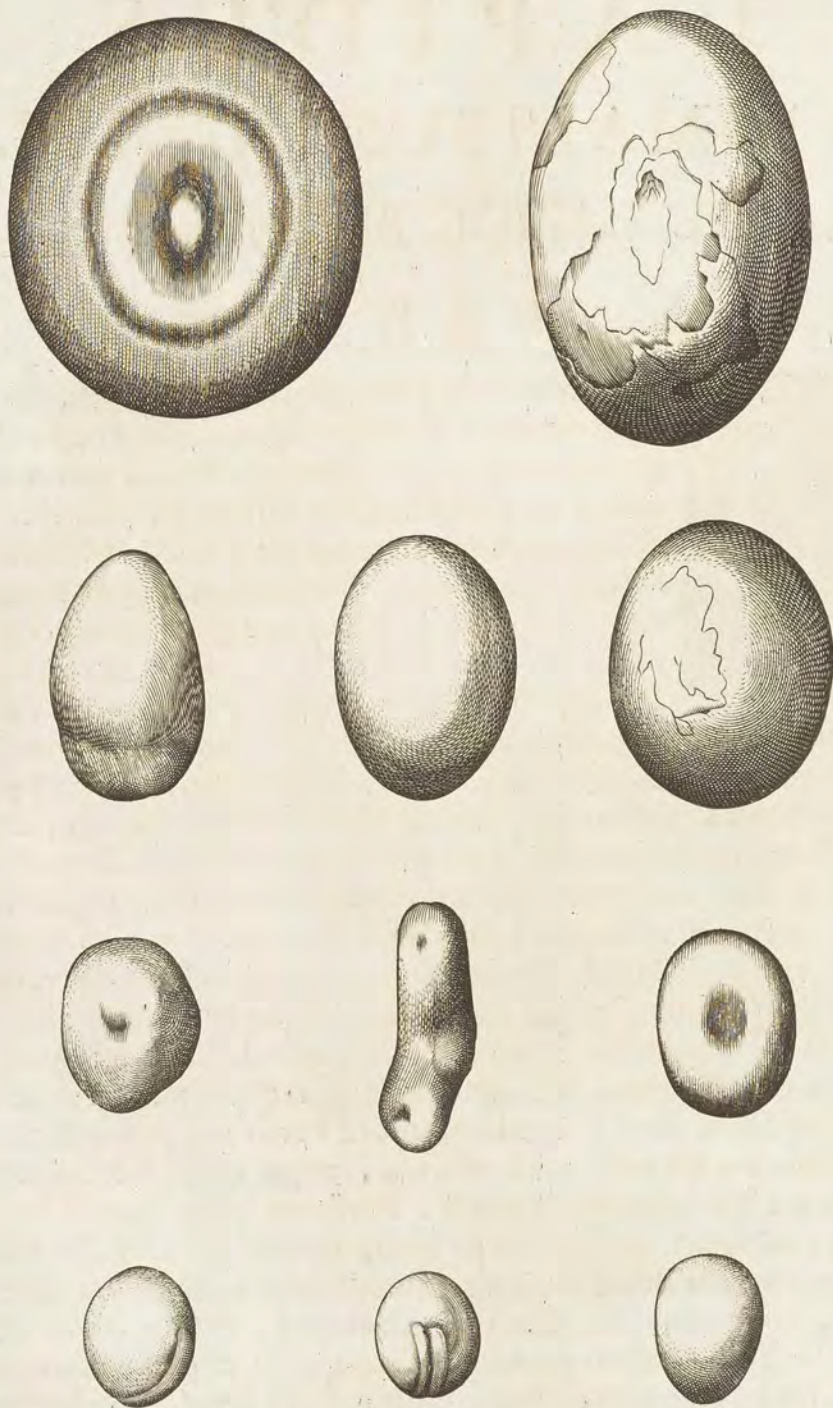
LAPIS BEZOARIUS
