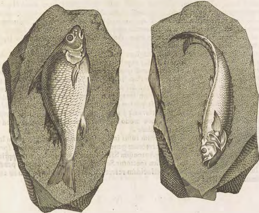
LAPIS ISLEBIANVS
