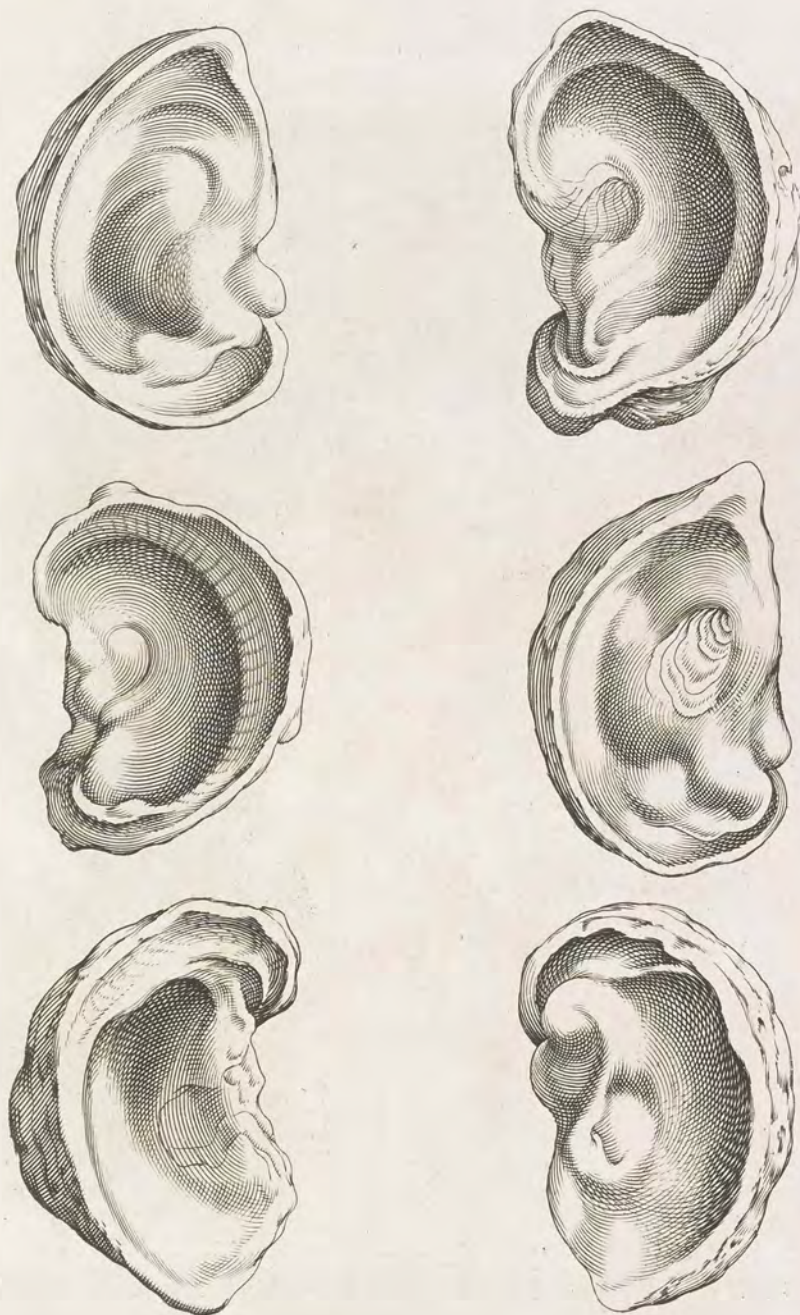
LAPIS AVRICVLARIS
