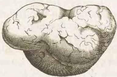
SILEX AVREVS
