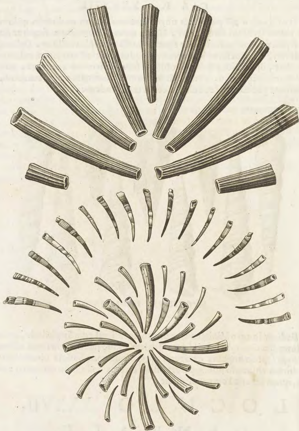
DENTALE
