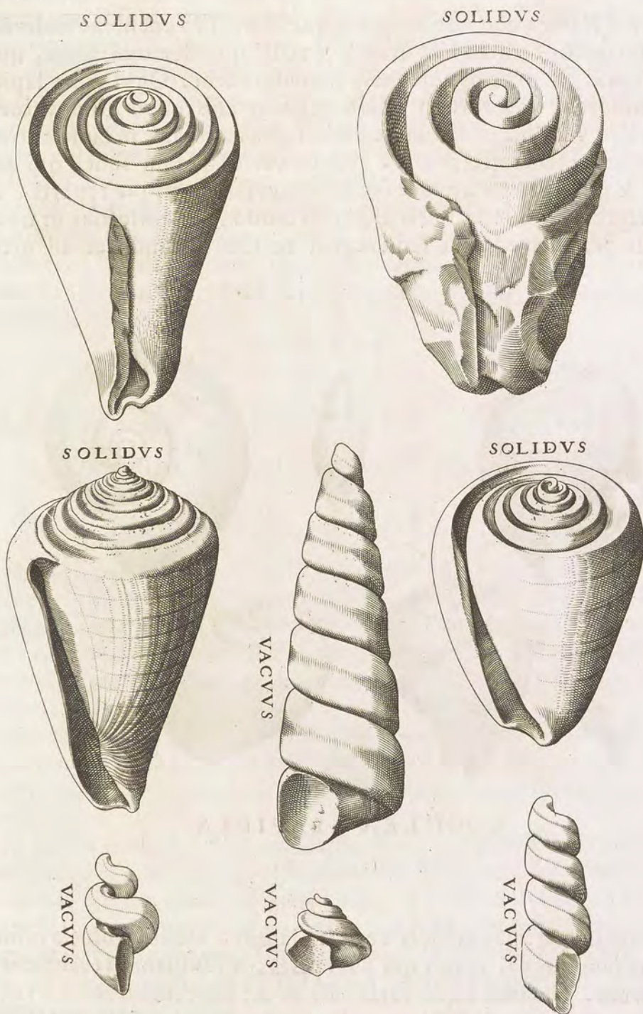
STROMBITES
