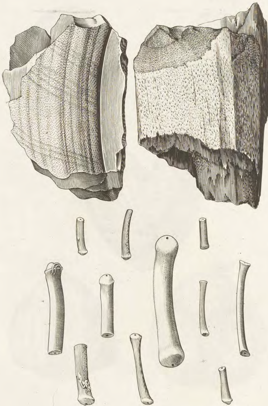
OSSA FOSSILIA
