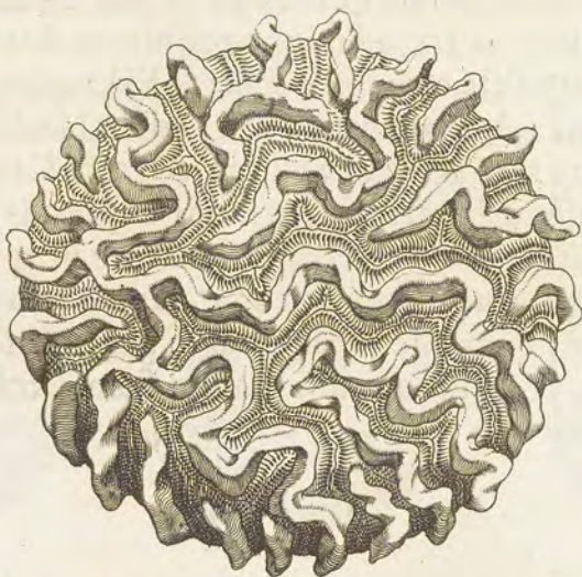
LAPIS LUMBRICATUS.
