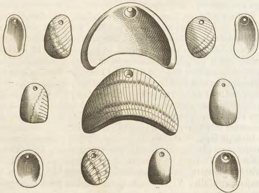
VNGVIS LAPIDEVS
