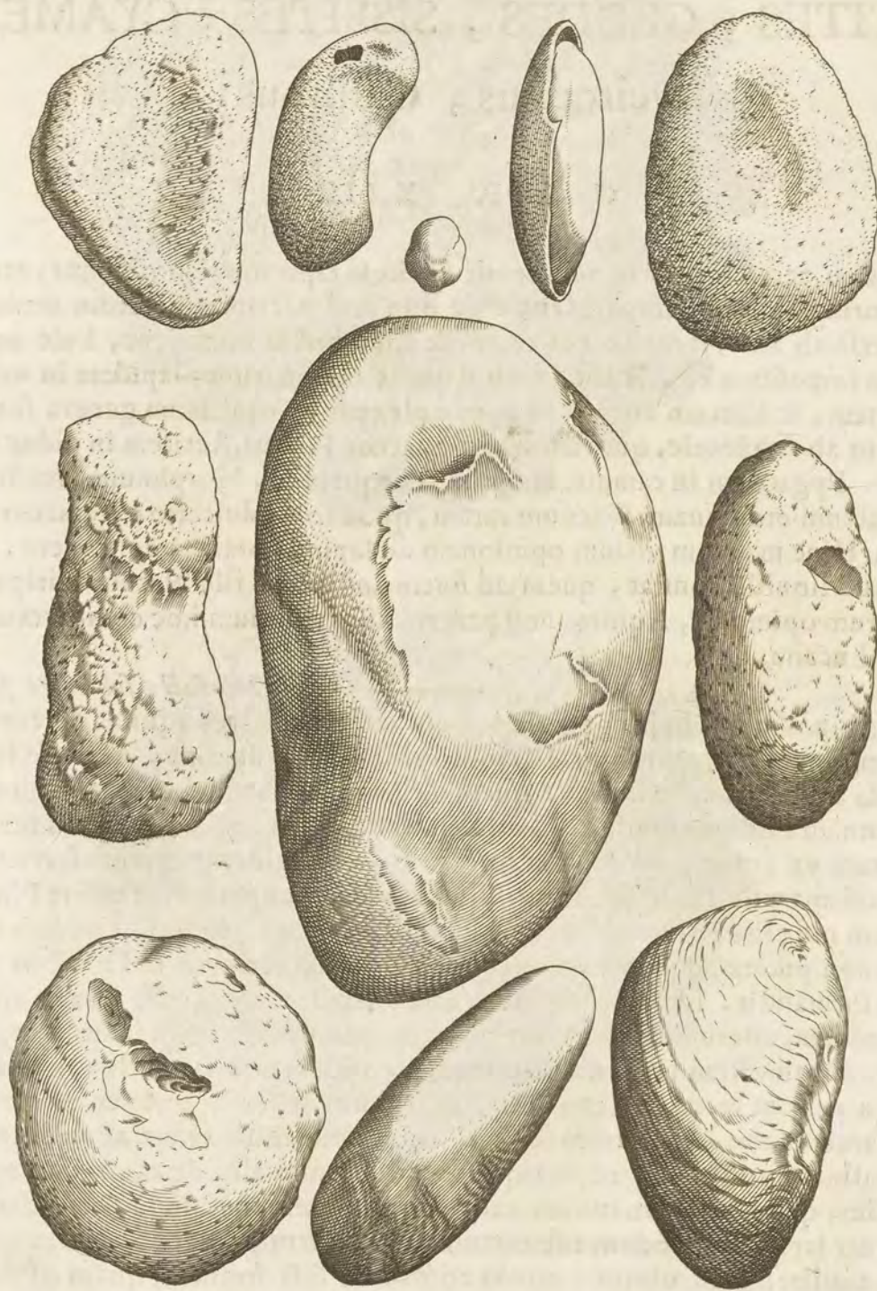
AETITES
