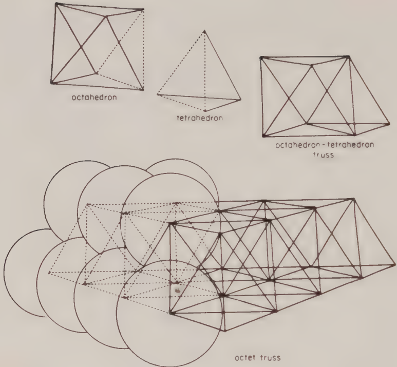
Fig. 420.01 Octet Truss .
