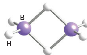
4 Diborane, \text{B}_2\text{H}_6
