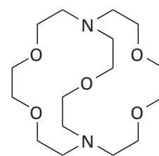
2 2.2.1-crypt
