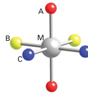
59 [MA 2 B 2 C 2 ]
