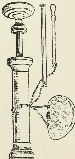
FIG. 36.—Fire Piston.
