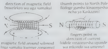
solenoids | solenoidi
