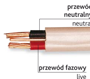
przewody | wires
