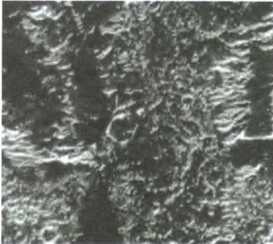
Mars Global Surveyor Hexagons
