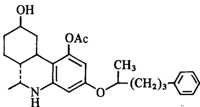
CP-44001-1 (Pfizer)
