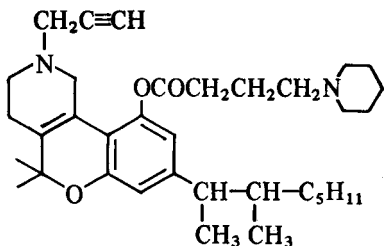
Nabitan (SP-106)
