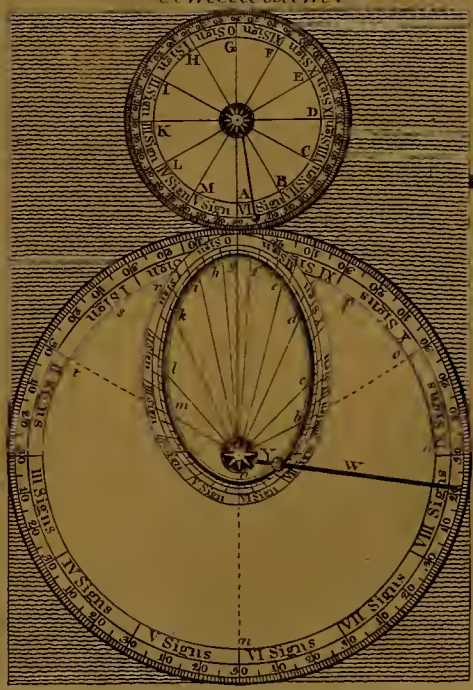
Fig. 216. Cometarium.
