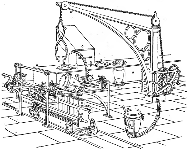
FIG. 1.—Furnace Apparatus.
