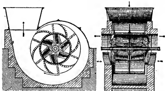
FIG. 19.—Capell Fan.
