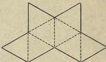
OCTAHEDRON.
