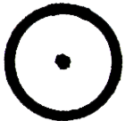
Solar Core (Sun)
