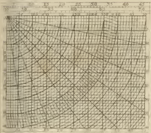
Fig. 5. Smical Quadrant.
