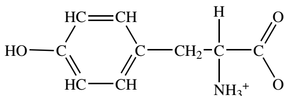
tyrosine
