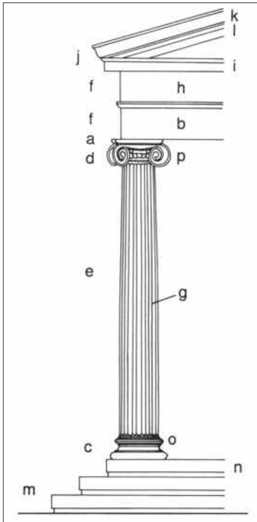
6.19 Main elements of the Ionic order: a) abacus; b) architrave; c) base; d) capital; e) column; f) entablature; g) fluting; h) frieze; i) horizontal cornice; j) pediment; k) sima; l) sloping cornice; m) steps or stereobate; n) stylobate; o) torus; p) volute
