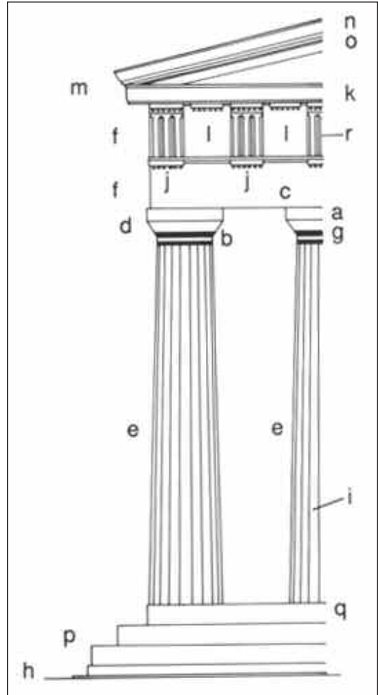
6.16 Main elements of the Doric order: a) abacus; b) annuli; c) architrave; d) capital; e) columns; f) entablature; g) echinus; h) euthynteria; i) fluting; j) guttae; k) horizontal cornice; l) metope; m) pediment; n) sima; o) slanting cornice; p) steps; q) stylobate; r) triglyph
